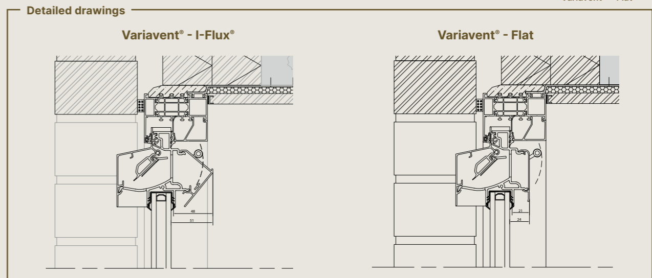
Variavent® - Flat
